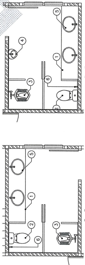
1.2.3 ห้องน้ำห้องงักที่ T4A SCALE 1 : 50 แสดงพื้นที่ของงบประมาณ
